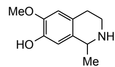
9. Salsolinol
