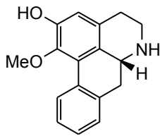
1. Asimilobine
