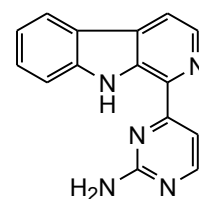
15. Annomontine
