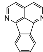
12. Canangine
