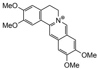
4. Pseudopalmatine
