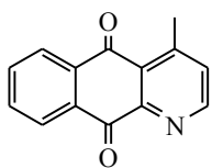
13. Cleistopholine
