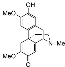
5. Sebiferine
